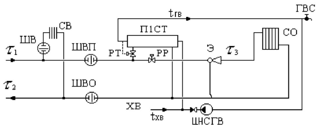
Рисунок 34 - МТП с параллельным подключением подогревателя ГВС и элеваторным присоединением СО
